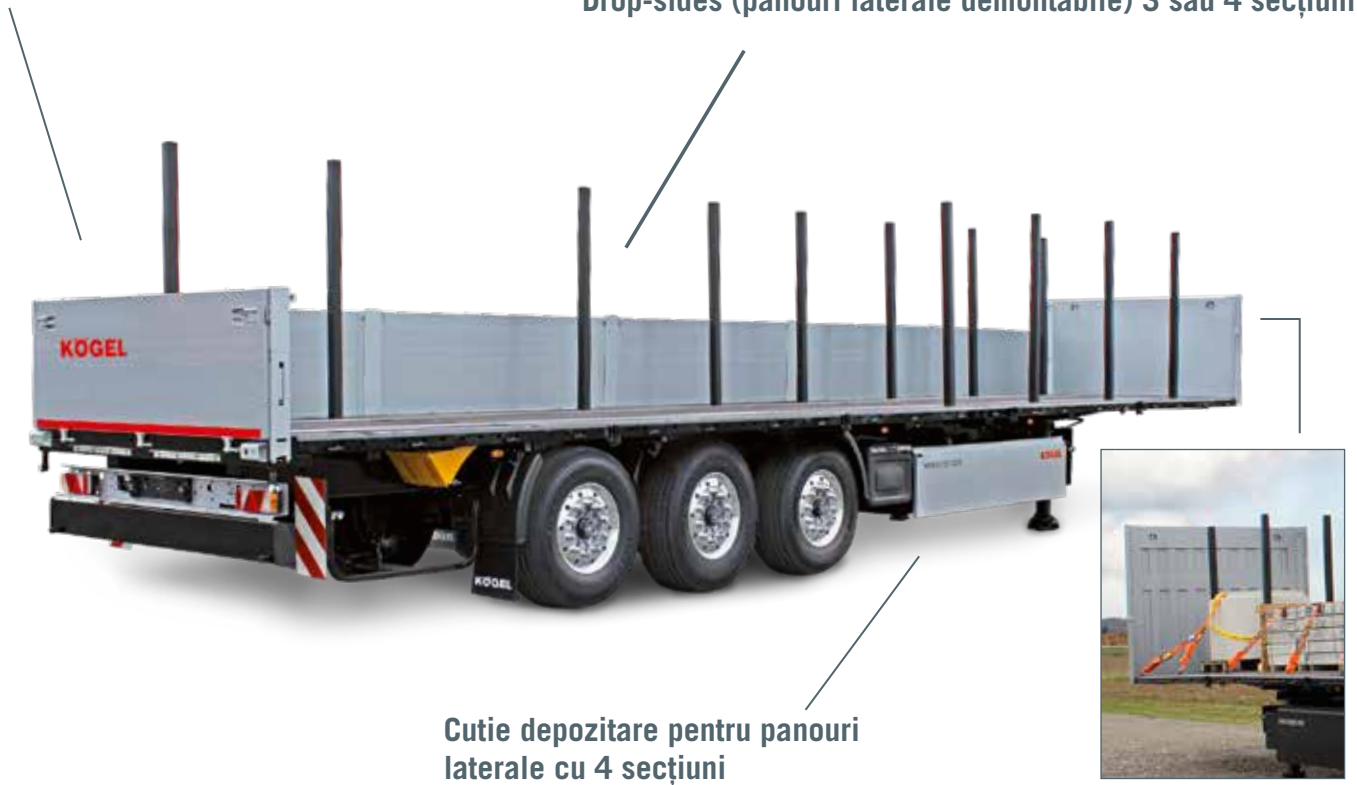
Panouri frontale din oțel sau aluminiu, cu înălțimi diferite
